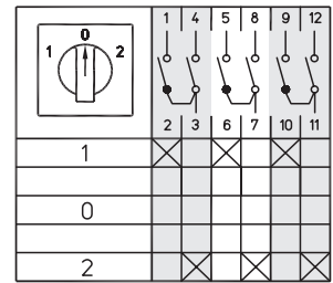
3-полюсные Схема 53
