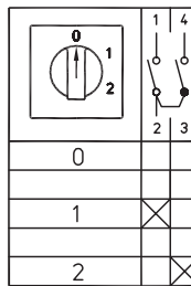
1-полюсные 2 позиции Схема 107
