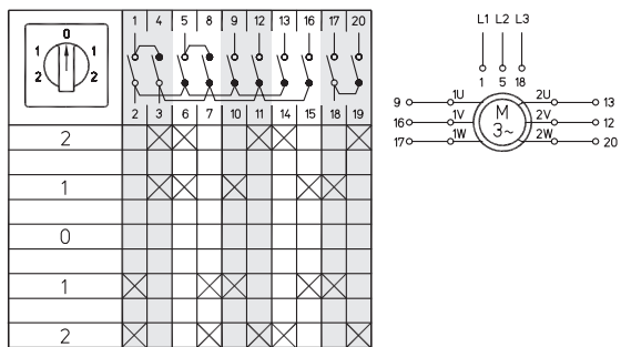
Двунаправленные Схема 23
