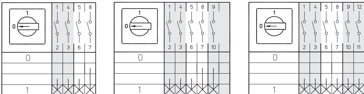
3 контакта с опережением 30°, 1 контакт с опережением 60° 4-полюсные Схема 272
