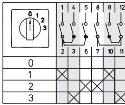
2-полюсные 3 позиции Схема 124
