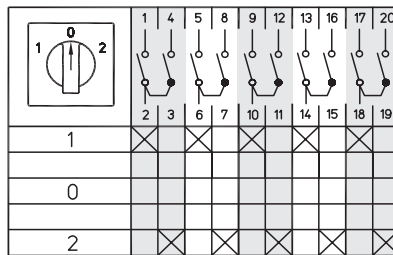
5-полюсные Схема 76
