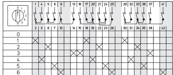
3-полюсные, 6 позиции Схема 139
