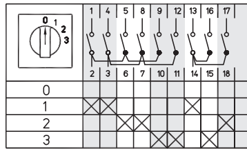
3-полюсные, 3 позиции Схема 136
