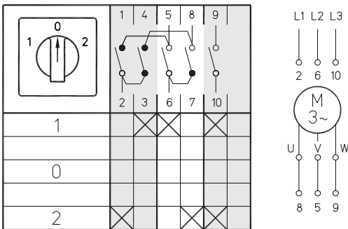
3-полюсные Схема 11
